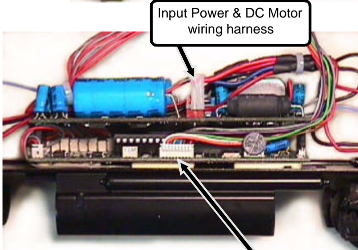
SwVol wiring harness
